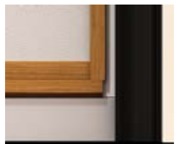
Устанавливаем нижний профиль для облицовки в стык с нижним профилем ворот, соблюдая технологический зазор в 1 мм до боковой крышки с каждой стороны
